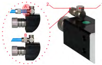
Abb. 3: Druckluftanschluss
