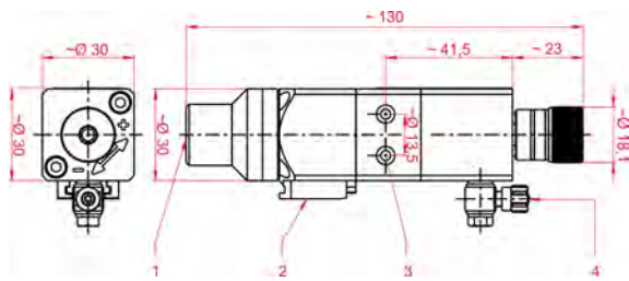
Abb. 8: Abmessungen Dosierventil EP-SV 295243
