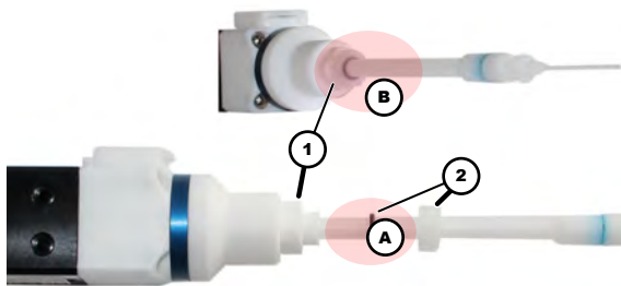
Abb. 4: Dosieranschluss bei Rotorspray
