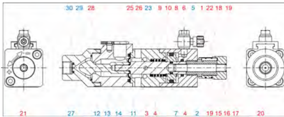
Abb. 6: Verschleiß- und Ersatzteile für Dosierventil EP-SV 295243
