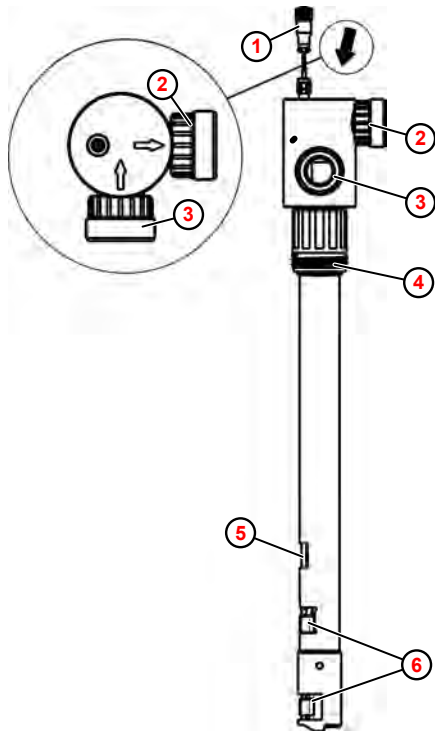
Abb. 1: Aufbau
