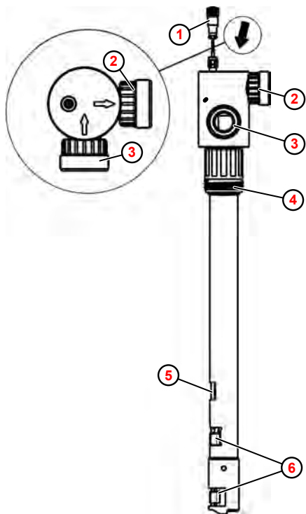
Fig. 1 : Construction
