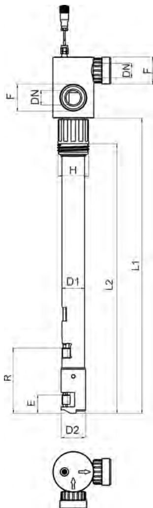
Fig. 7 : Dimensions de la lance d'aspiration
