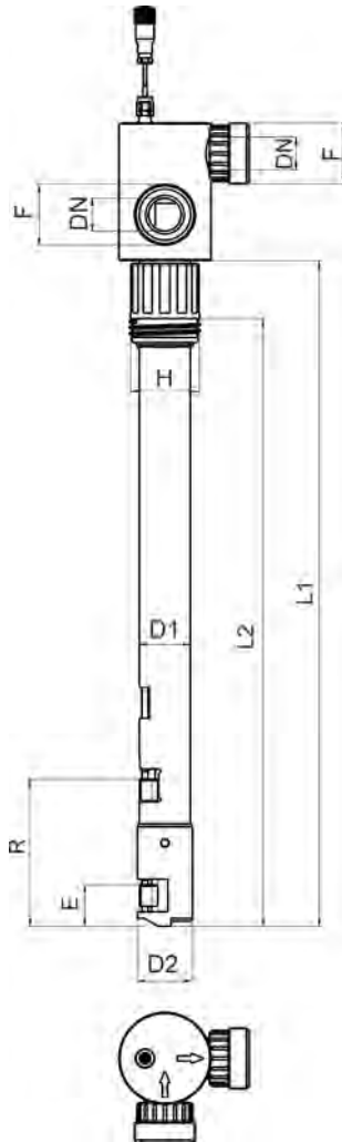
Abb. 7: Abmessungen Sauglanze
