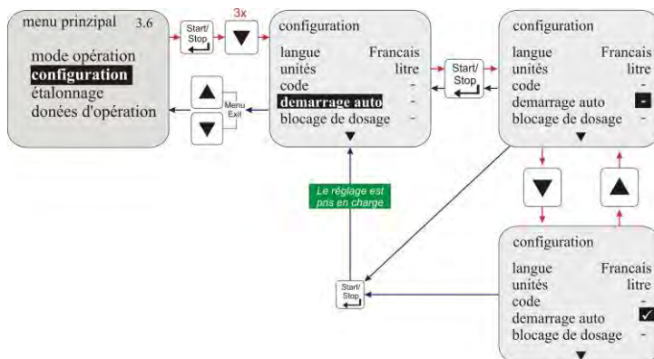
Fig. 10.20 Configuration / Demarrage auto / Sélectionner
