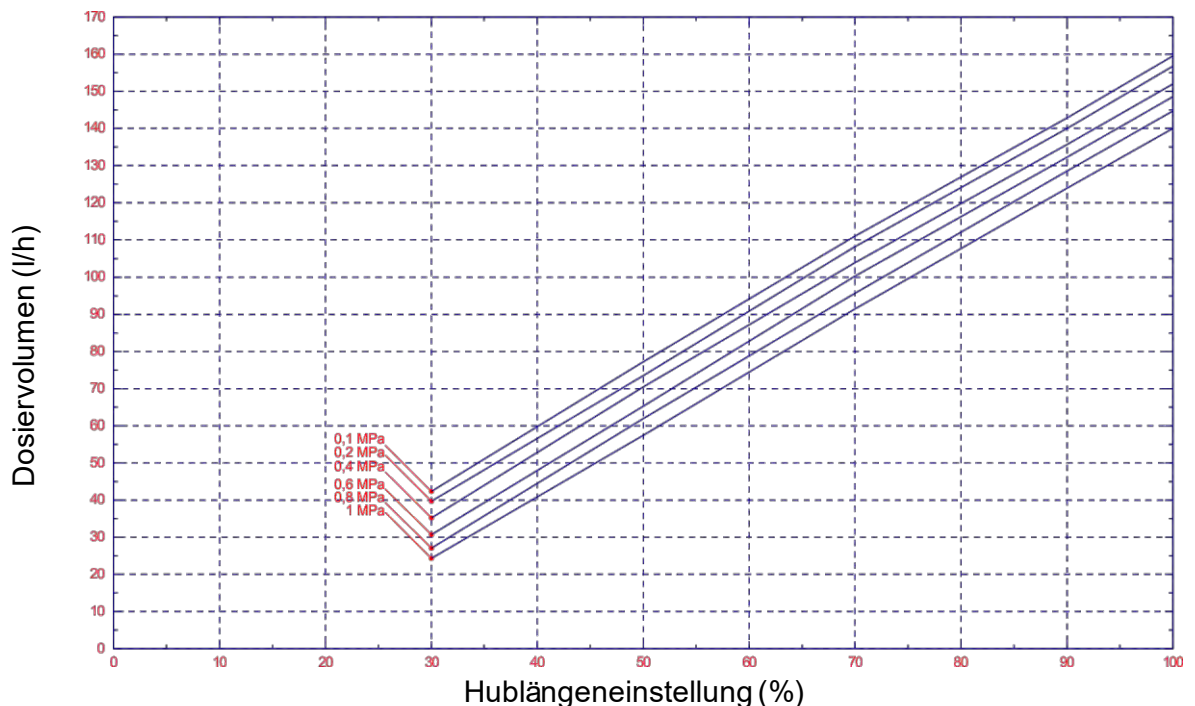
Abb. 14.3 Förderleistung Typ 01400 / 1 MPa (10 bar)
