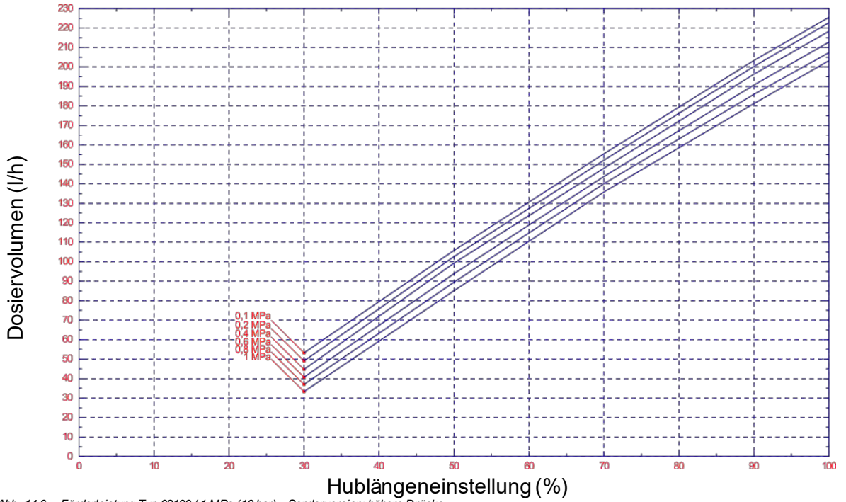
Abb. 14.6 Förderleistung Typ 02100 / 1 MPa (10 bar) - Sonderversion: höhere Drücke
