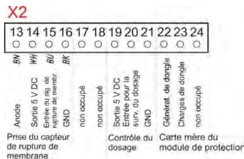
Fig. 7.25 Affectation des broches connecteur - Bornier X2
