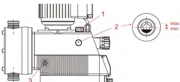
Abb. 11.5 Getriebeölwechsel
