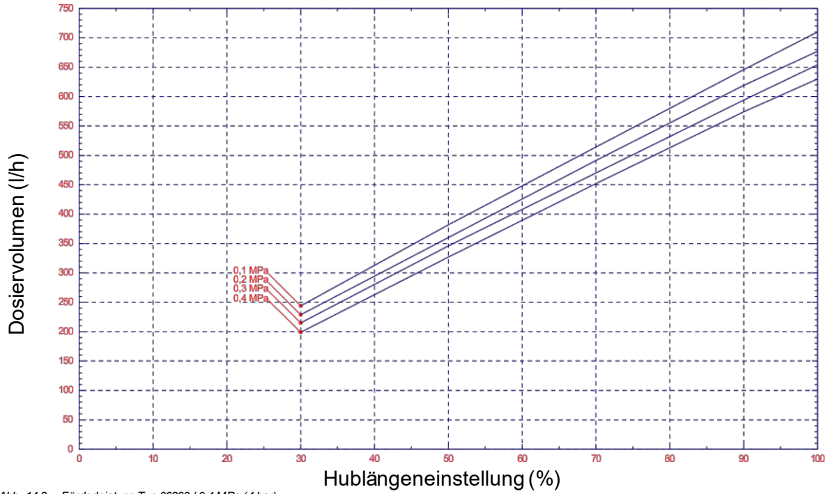
Abb. 14.8 Förderleistung Typ 06300 / 0,4 MPa (4 bar)
