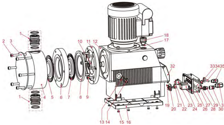
Abb. 13.1 Verschleiß und Ersatzteile
