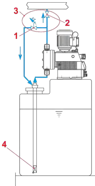
Abb. 6.1 Einbauschema
