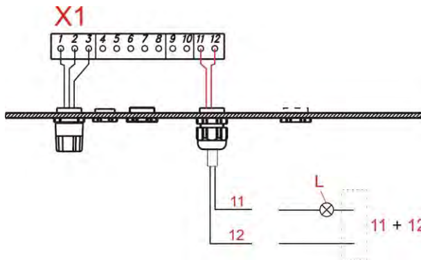
Abb. 7.24 Installation Hubsignalausgang
