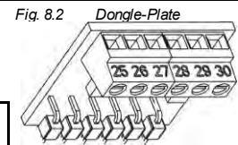
Fig. 8.2 Dongle-Plate
