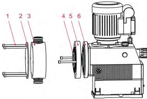
Fig. 11.4 Remplacement de la tête de pompe et de la membrane
