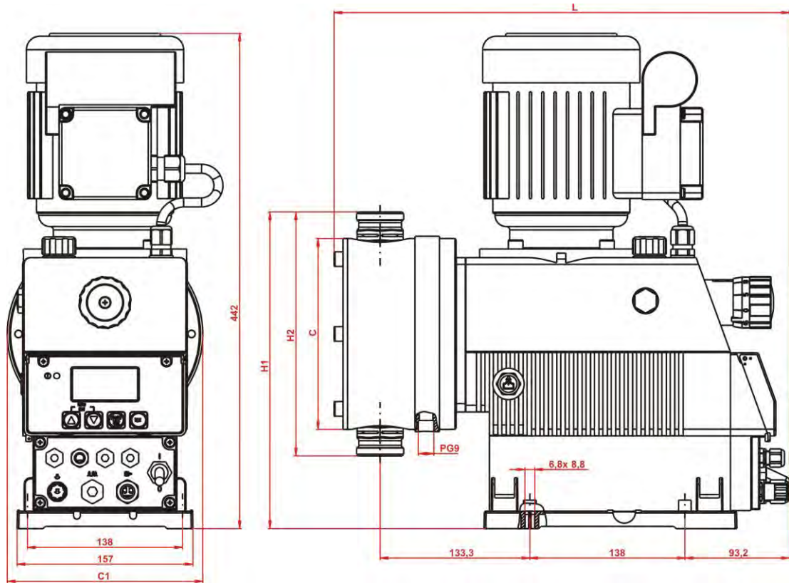
Fig. 14.1 Dimensions
