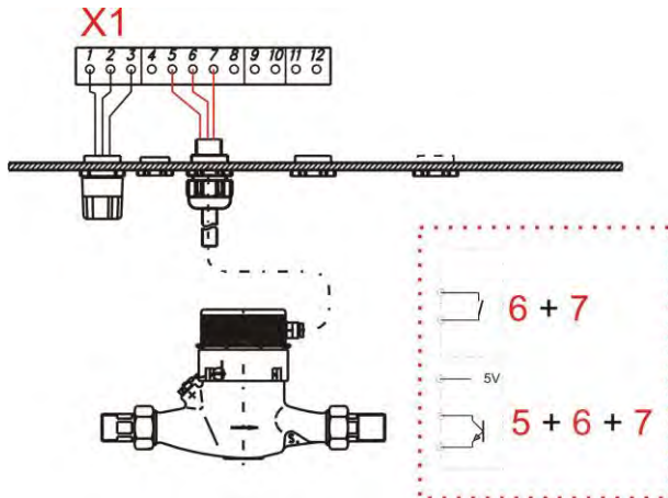
Abb. 7.20 Installation Impulsansteuerung (Wasserzähler)
