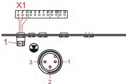
Abb. 7.18 Anschlussbelegung Steckplatz I
