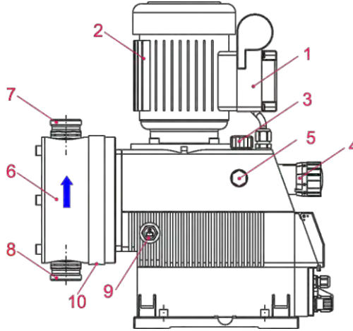
Fig. 5.2 EMP IV E60 (latéral)
