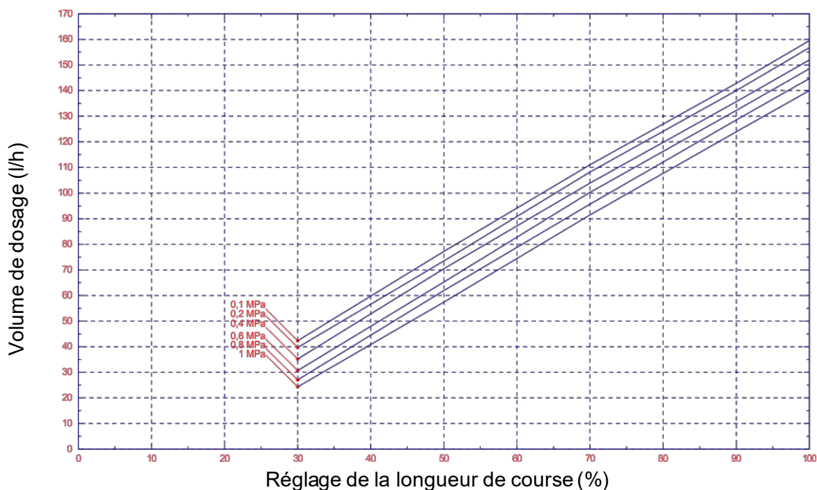
Fig. 14.3 Performance de débit - type 01400 / 1 MPa (10 bar)
