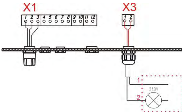
Abb. 7.30 Installation Niveau- bzw. Störmeldeausgang
