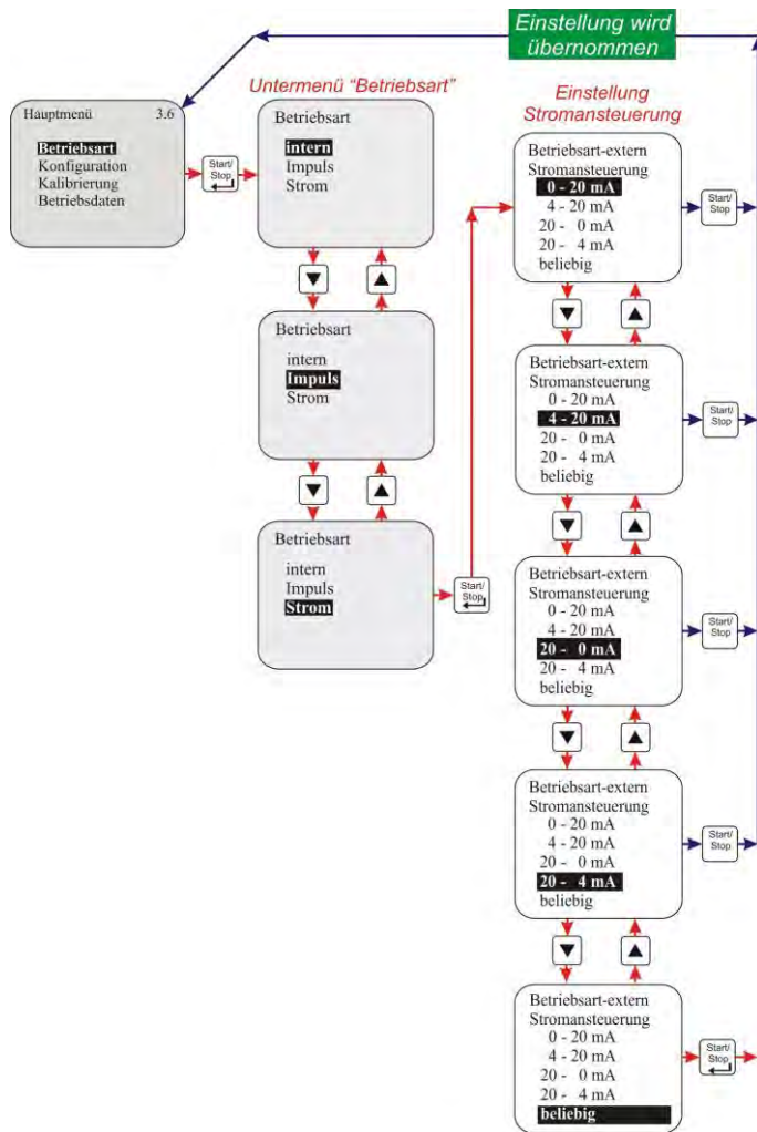
Abb. 10.11 Betriebsart / Strom / Auswählen
