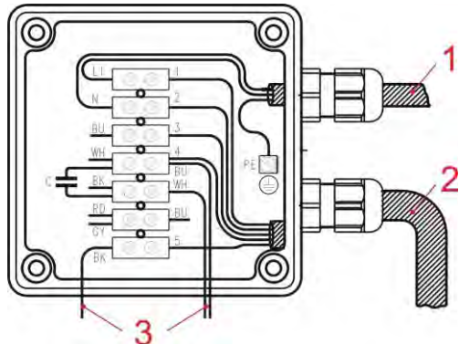
Abb. 7.14 Netzanschluss
