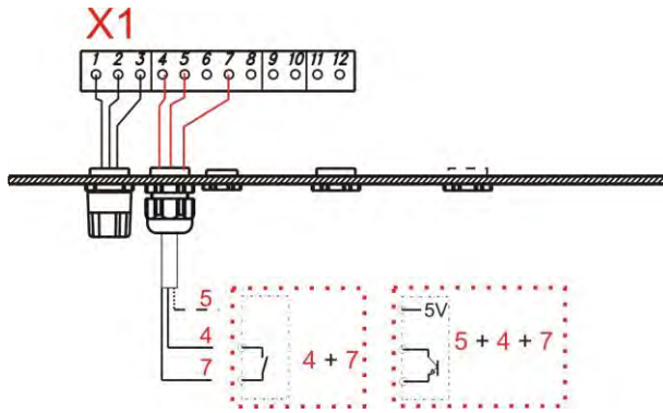
Abb. 7.23 Installation Chargensteuerung
