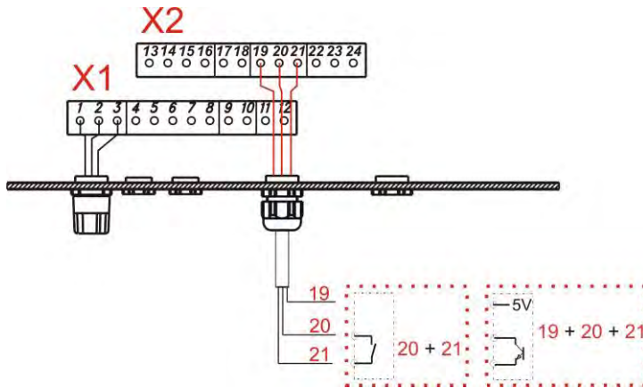
Abb. 7.28 Installation Dosierüberwachung
