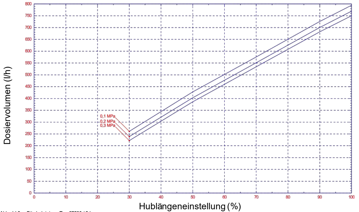
Abb. 14.9 Förderleistung Typ 07500 / 3 bar
