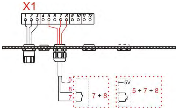
Abb. 7.22 Installation Ansteuerung über Dosiersperre
