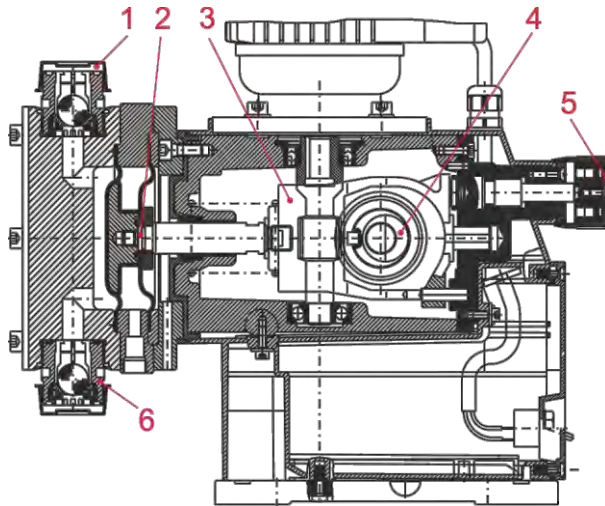
Abb. 4.1 Funktionsbeschreibung – Mechanische Funktionen
