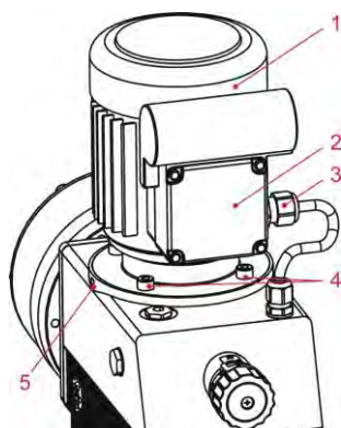
Fig. 11.6 Remplacement du moteur
