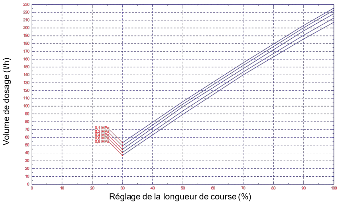
Fig. 14.5 Performance de débit - type 02100 / 0,8 MPa (8 bar)
