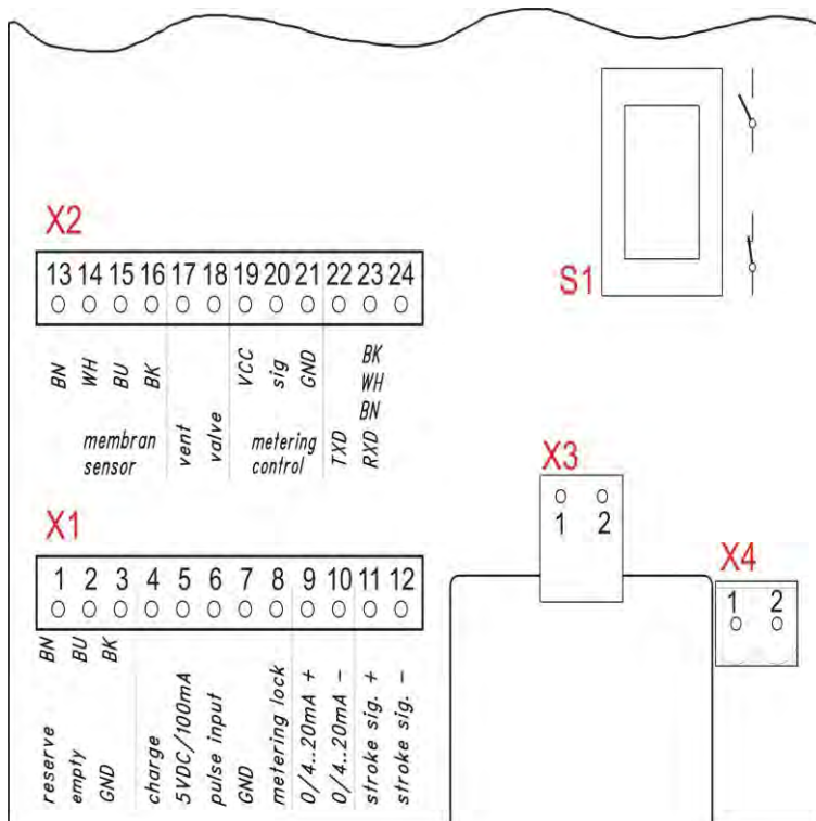
Fig. 7.16 Aperçu – Borne plate
