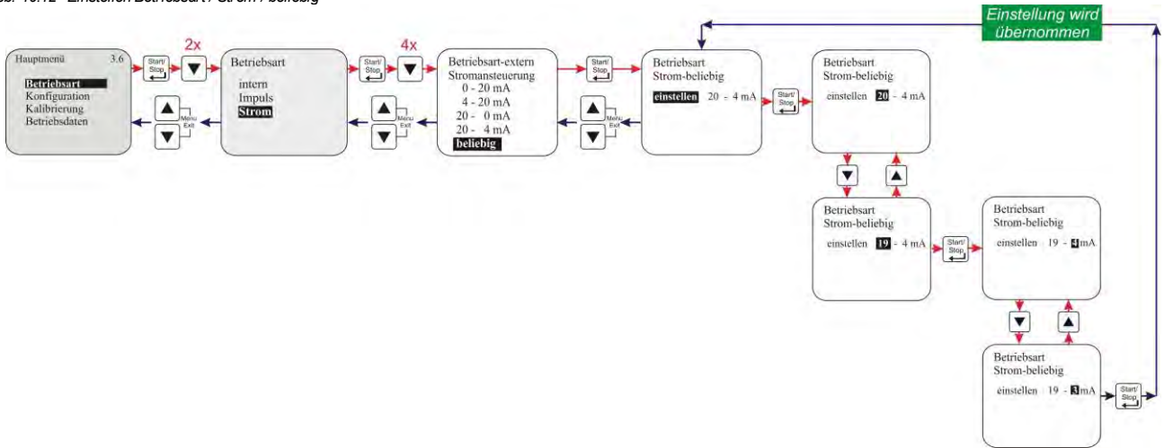
Abb. 10.12 Einstellen Betriebsart / Strom / beliebig
