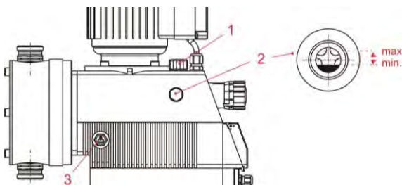
Fig. 11.5 Vidange de l'huile d'engrenage
