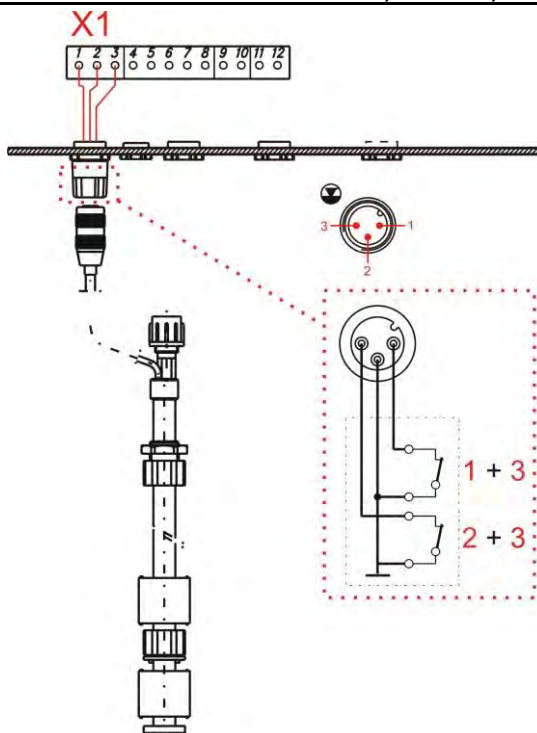
Abb. 7.19 Installation Sauglanze mit Niveuvorwarnung und Leermeldung
