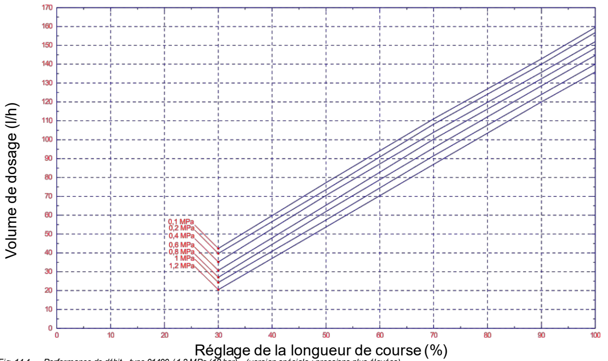
Fig. 14.4 Performance de débit - type 01400 / 1,2 MPa (12 bar) - (version spéciale : pressions plus élevées)
