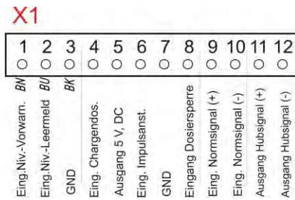
Abb. 7.17 Klemmleiste X1
