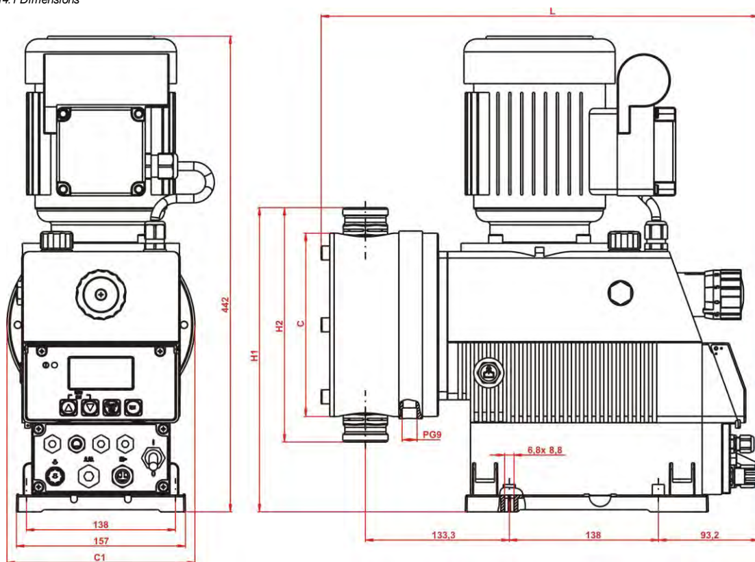
Fig. 14.1 Dimensions
