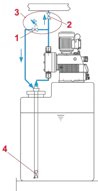
Fig. 6.1 Schéma de montage
