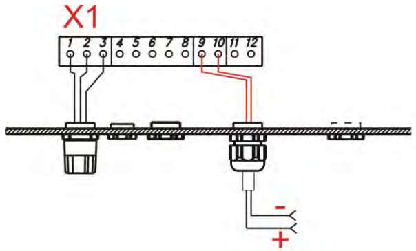
Fig. 7.21 Installation de la commande du signal normalisé
