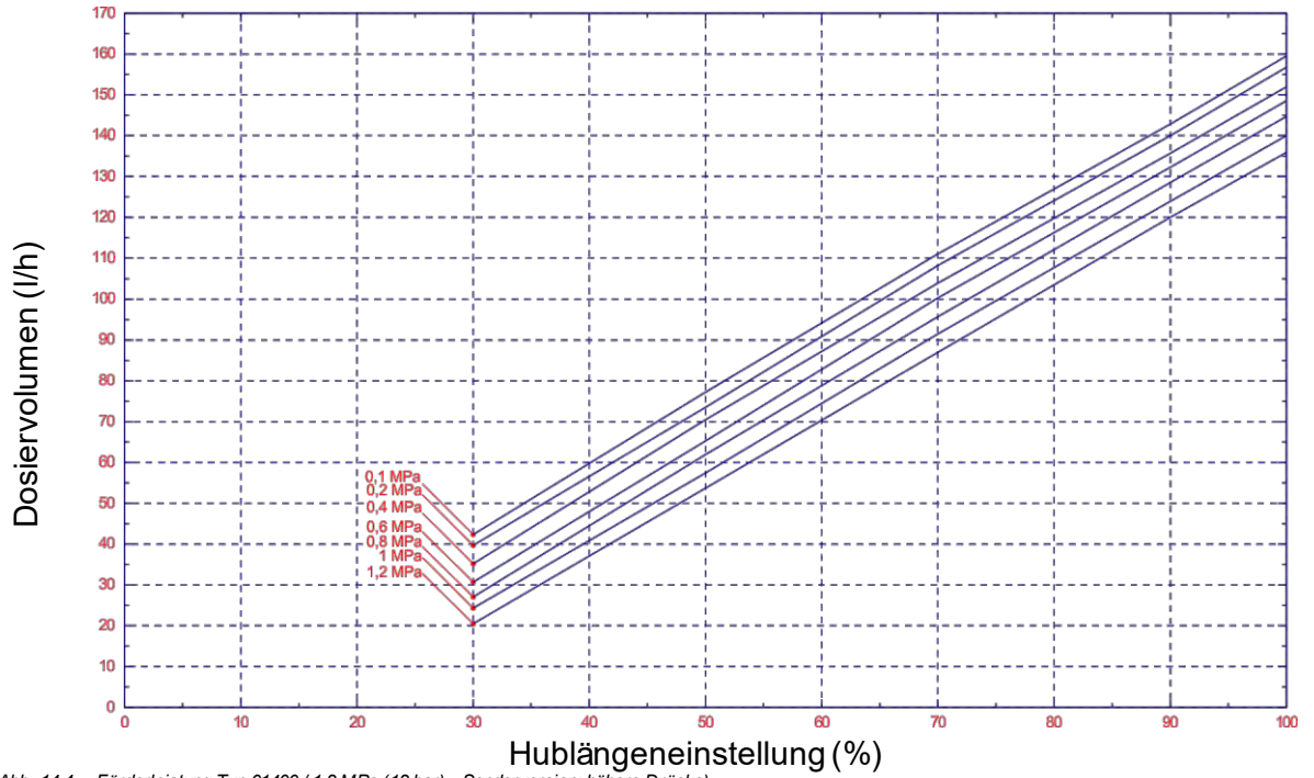
Abb. 14.4 Förderleistung Typ 01400 / 1,2 MPa (12 bar) - Sonderversion: höhere Drücke
