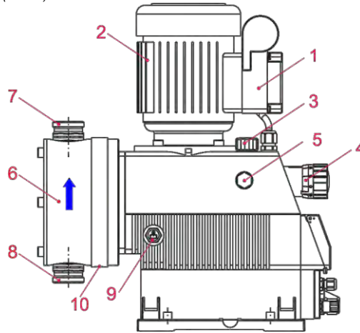
Abb. 5.2 EMP IV E60 (seitlich)
