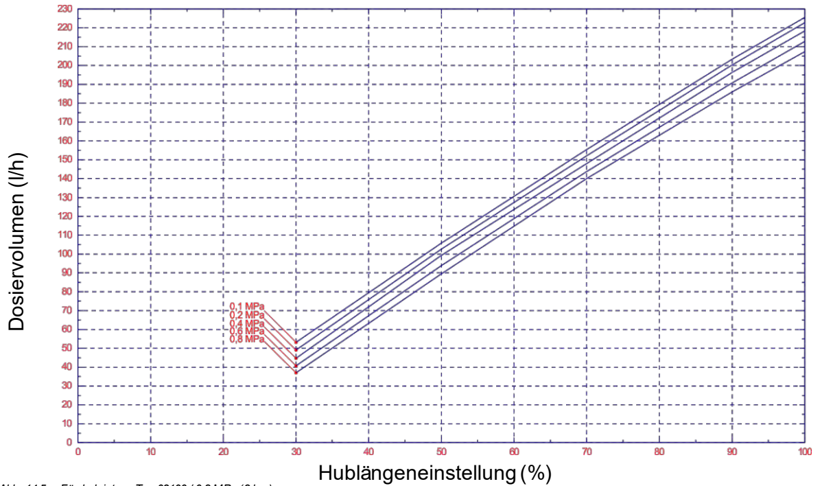
Abb. 14.5 Förderleistung Typ 02100 / 0,8 MPa (8 bar)
