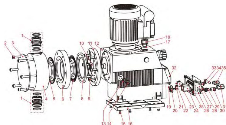
Fig. 13.1 Pièces d'usure et pièces détachées
