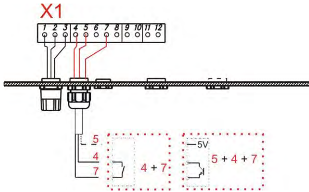
Fig. 7.23 Installation de la fonction de charge
