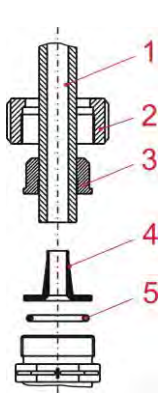
Abb. 7.13 Anschluss der Saug- und Dosierleitung mit Kegelteil
