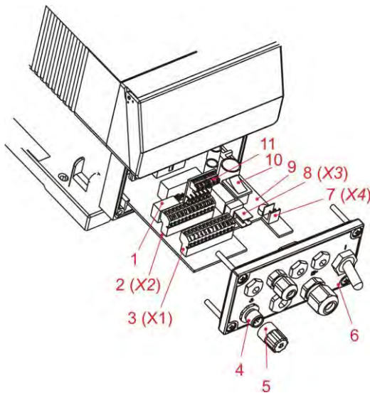
Abb. 7.15 Übersicht Steuerplatine
