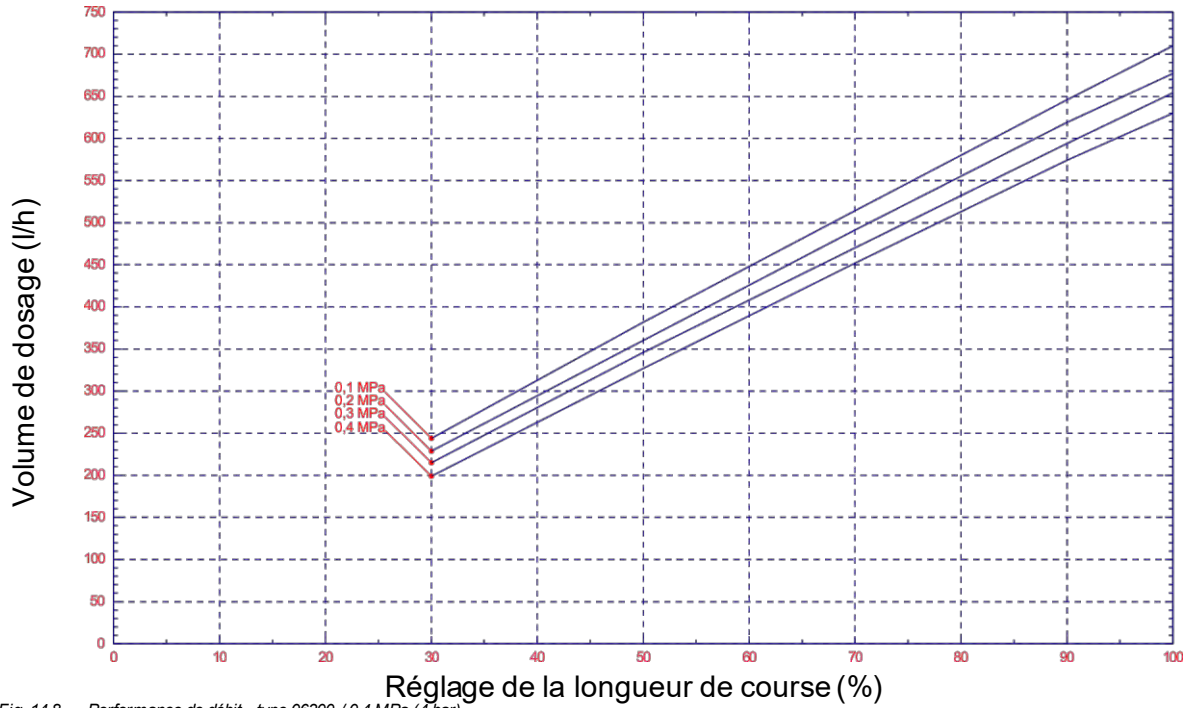
Fig. 14.8 Performance de débit - type 06300 / 0,4 MPa (4 bar)
