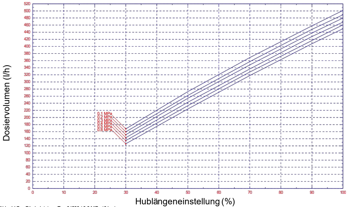
Abb. 14.7 Förderleistung Typ 04500 / 0,6 MPa (6 bar)
