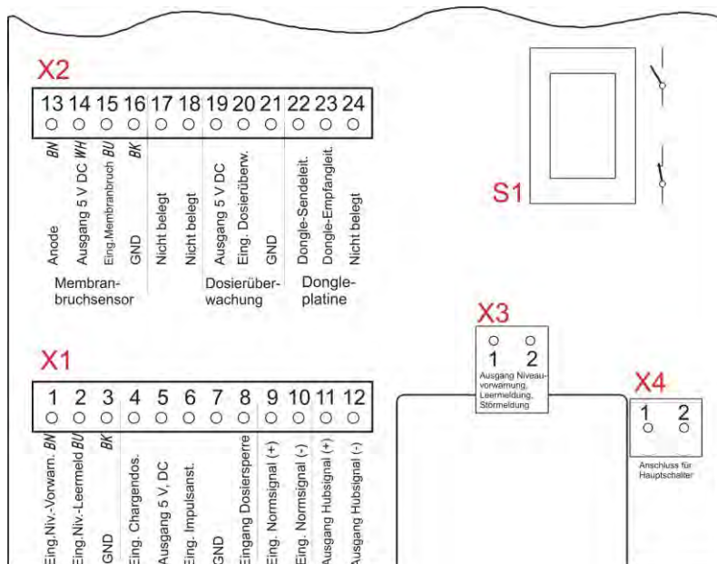
Abb. 7.16 Klemmleistenübersicht
