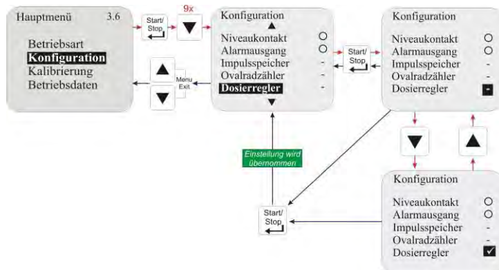
Abb. 10.29 Konfiguration / Dosierregler / Auswählen
