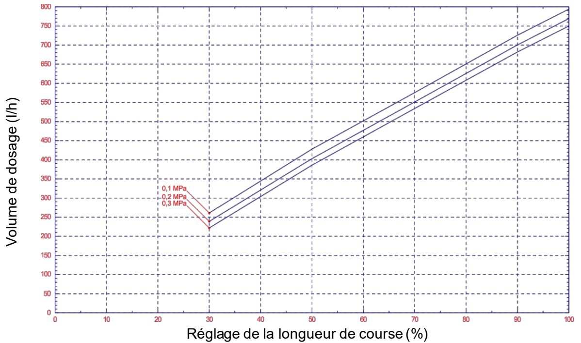
Fig. 14.9 Performance de débit - type 07500 / 0,3 MPa (3 bar)
