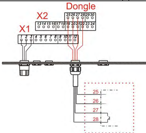
Fig. 8.2 Installation du compteur à roues ovales
