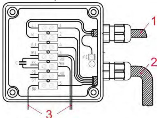
Fig. 7.14 Connexion au réseau
