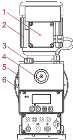
Abb. 5.1 EMP IV E60 (vorne)
