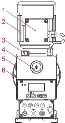
Fig. 5.1 EMP IV E60 (Front)
