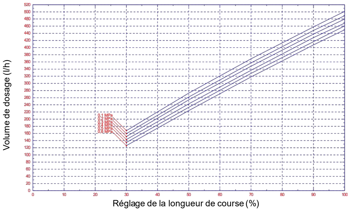
Fig. 14.7 Performance de débit - type 04500 / 0,6 MPa (6 bar)
