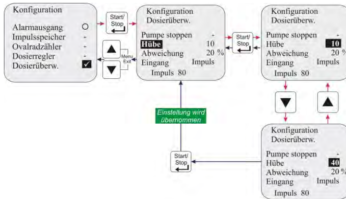
Abb. 10.36 Konfiguration / Dosierüberwachung / Hube
