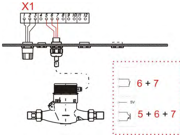
Fig. 7.20 Installation de la commande d'impulsion (compteur d'eau)
