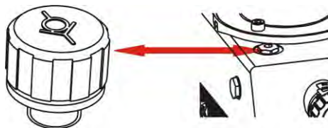
Abb. 9.7 Öleinfüllöffnung
