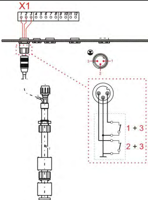
Fig. 7.19 Installation de la lance d'aspiration avec pré-avertissement de niveau et signalisation d'état vide
