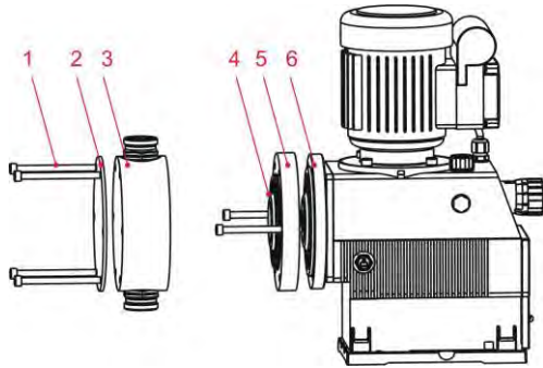
Abb. 11.4 Austausch des Pumpenkopfes und der Membrane
