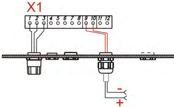
Abb. 7.21 Installation Normsignal Ansteuerung
