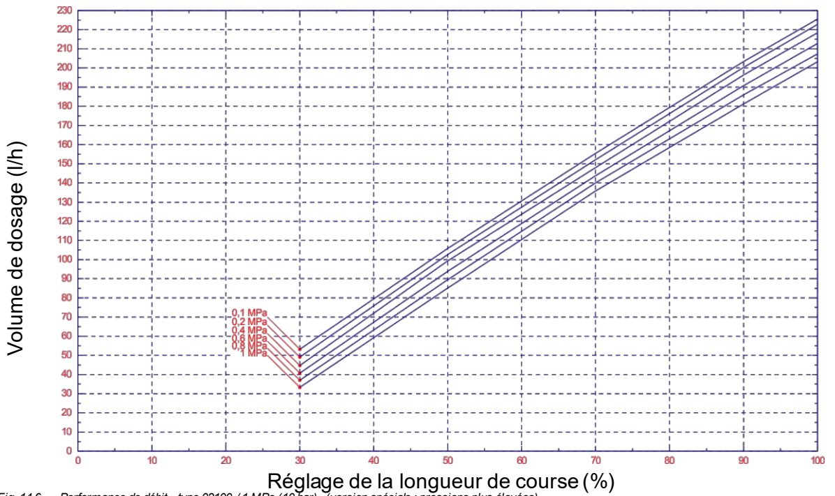
Fig. 14.6 Performance de débit - type 02100 / 1 MPa (10 bar) - (version spéciale : pressions plus élevées)
