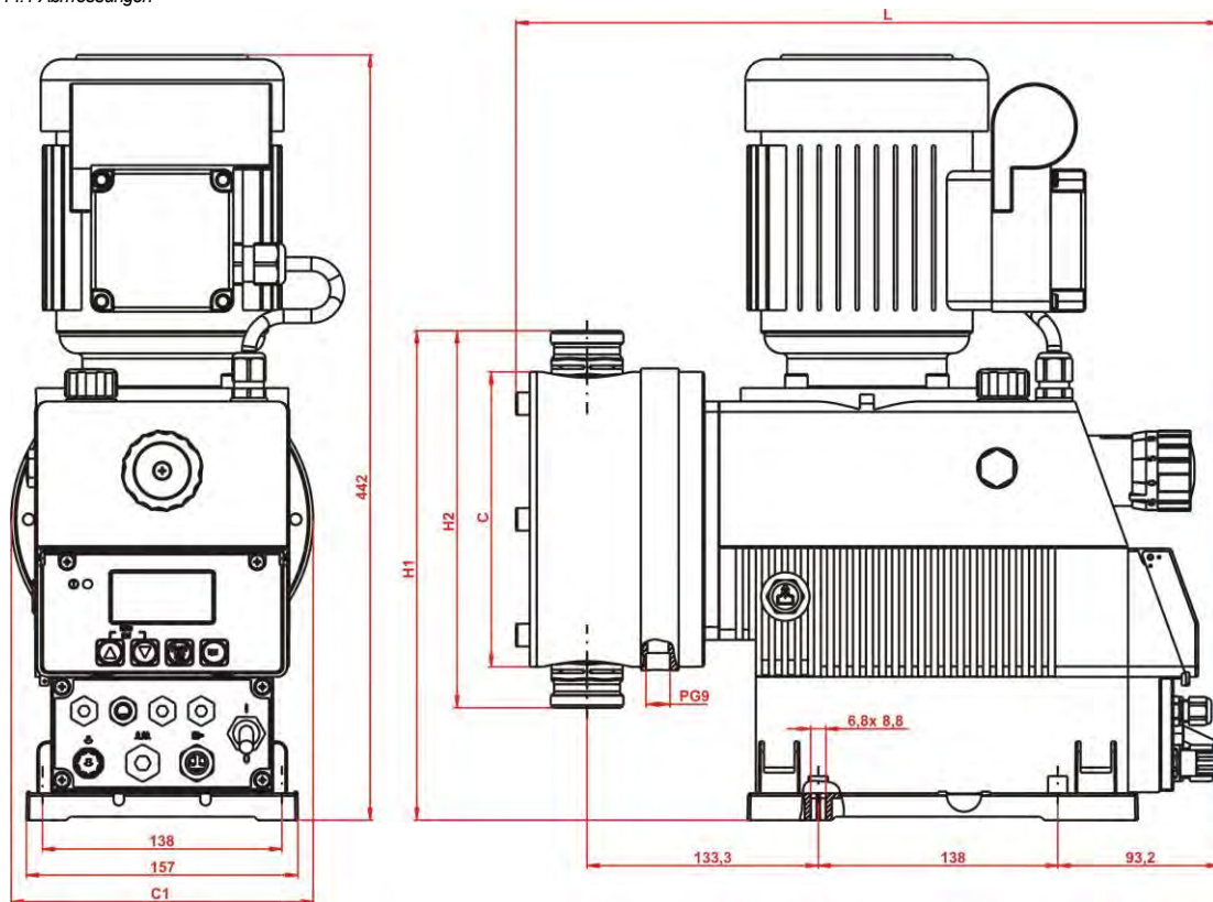
Abb. 14.1 Abmessungen
