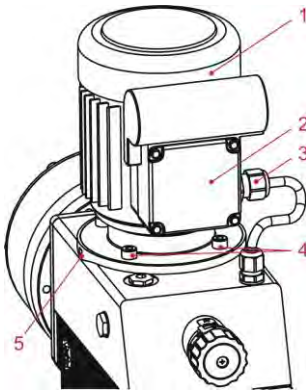
Abb. 11.6 Motor wechseln
