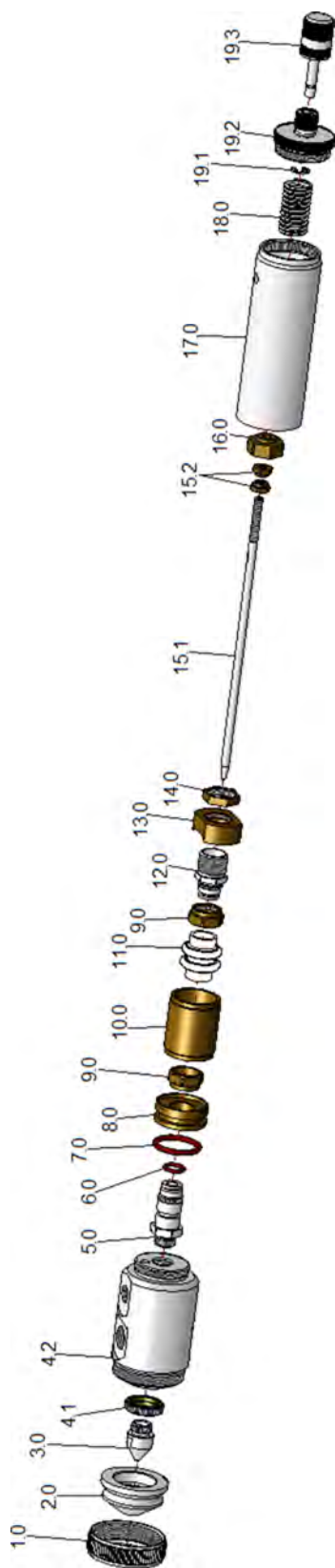
Abb. 8: Ersatzteile
